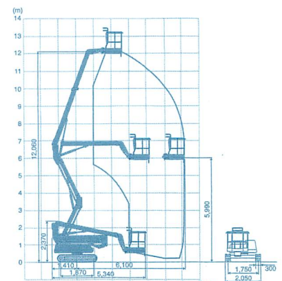
作業半径図 (HF-120)
